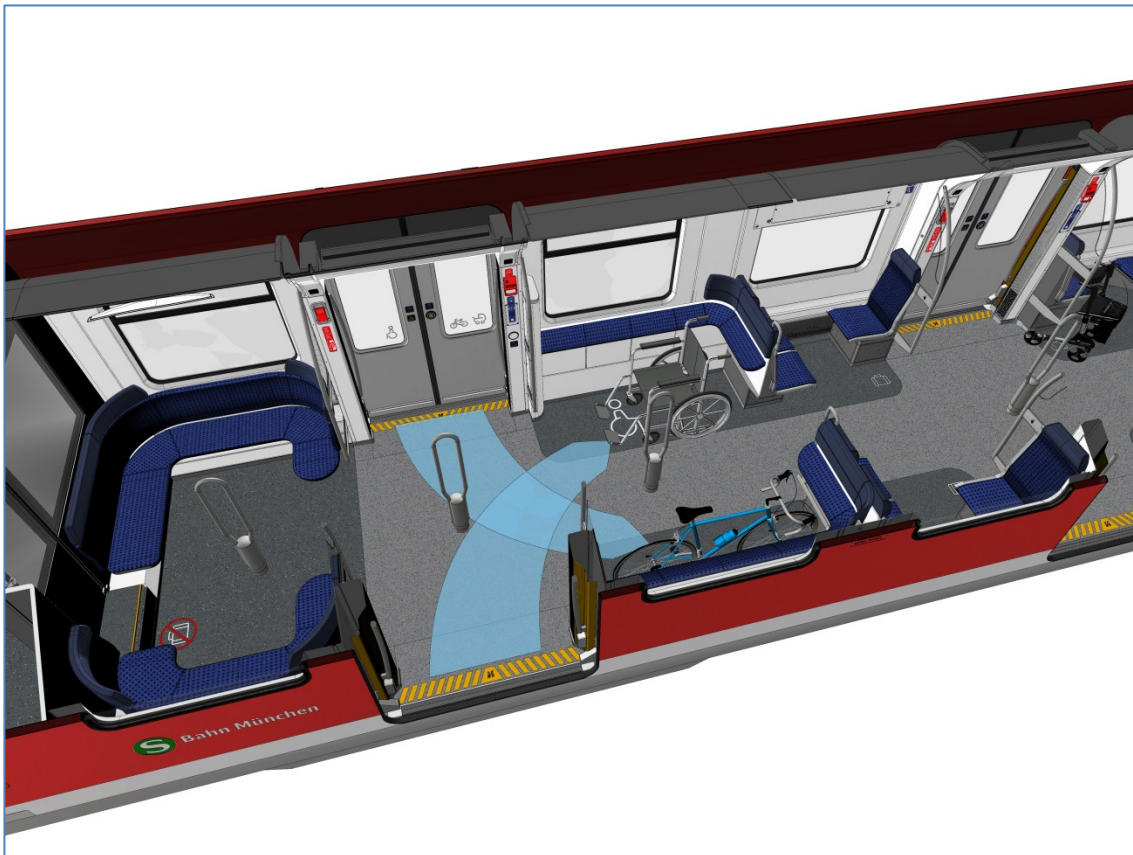
Abb. 105: ET423 Modernisierung – Gruppen- und Mehrzweckbereich
